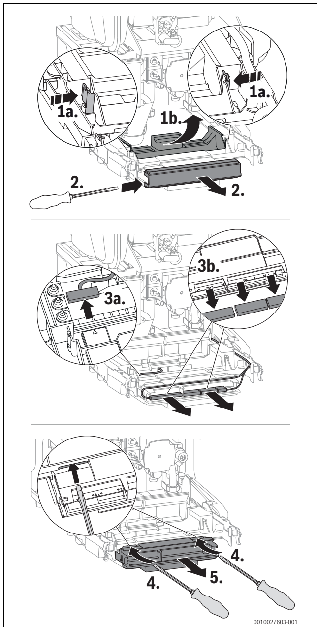
Fig. 78 Rimozione del dispositivo di controllo
