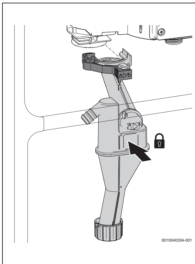
Fig. 83 Applicazione del sifone per la condensa
