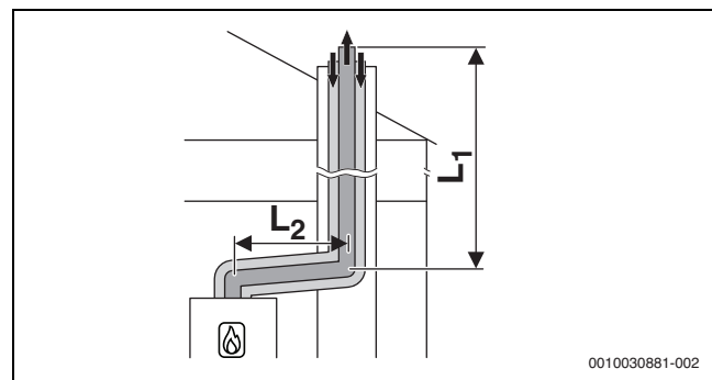
Fig. 12 Condotto di aspirazione aria comburente/evacuazione prodotti della combustione concentrico secondo C 33x nel cavedio
