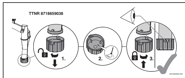
Fig. 80 Pulizia del dispositivo di ritenzione impurità
