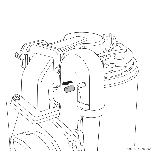
Fig. 47 Manicotto di misurazione sul miscelatore
