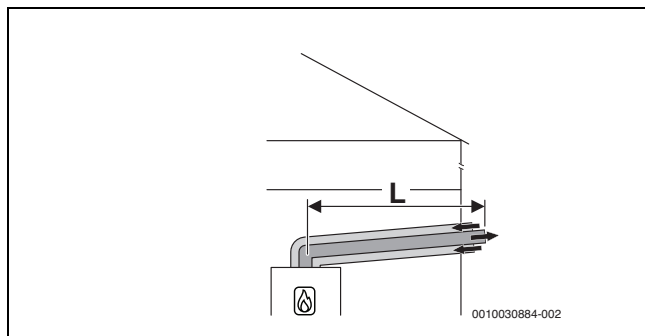
Fig. 10 Condotto di aspirazione aria comburente/evacuazione pdc orizzontale concentrico secondo C 13x attraverso la parete esterna
