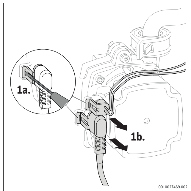
Fig. 66 Scollegamento del connettore dal circolatore riscaldamento
