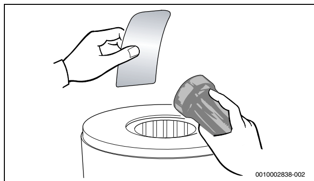
Fig. 62 Controllo della presenza di residui nello scambiatore primario
