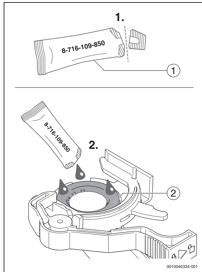
Fig. 82 Ingrassaggio della guarnizione
