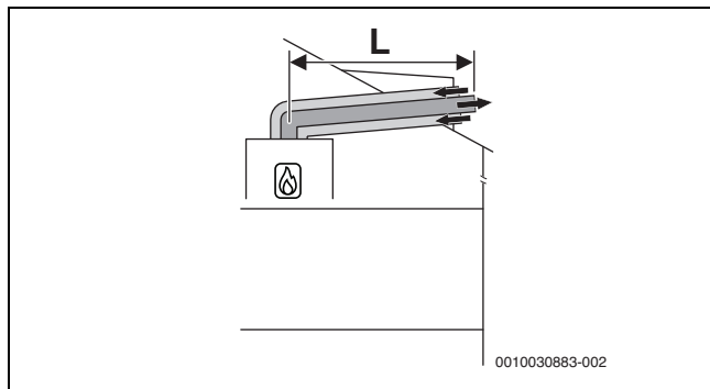
Fig. 11 Condotto di aspirazione aria comburente/evacuazione prodotti della combustione orizzontale concentrico secondo C 13x attraverso il tetto
