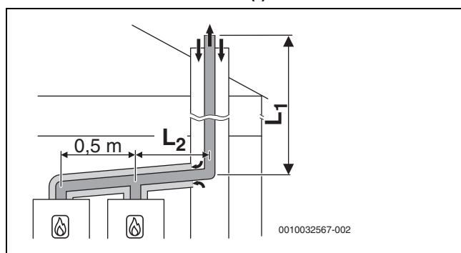
Fig. 27 Impianto a cascata con 2 apparecchi: sistema di aspirazione aria/evacuazione dei prodotti della combustione rigido secondo C_{93x} nel cavedio e condotto di aspirazione aria comburente/evacuazione prodotti della combustione concentrico nel luogo di posa
