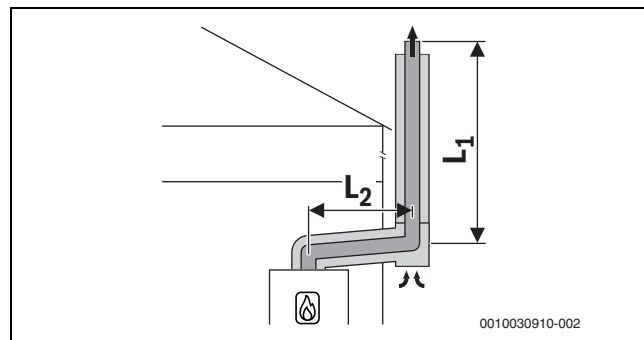
Fig. 17 Condotto di aspirazione aria comburente/evacuazione prodotti della combustione concentrico secondo C53x sulla parete esterna
