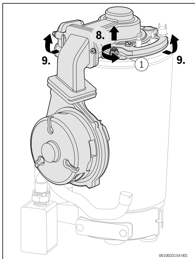
Fig. 52 Rimozione del coperchio del bruciatore con ventilatore e miscelatore
