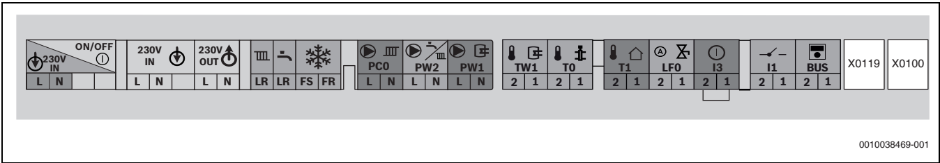
Fig. 40 Morsettiera per accessorio esterno
