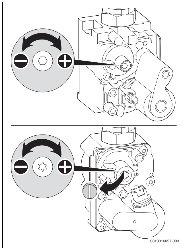
Fig. 45 Taratura della valvola del gas
