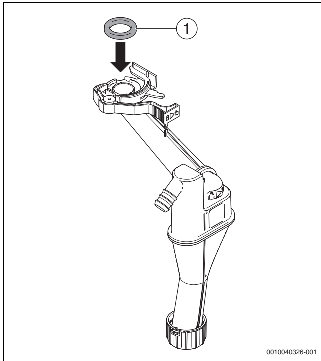
Fig. 81 Applicazione di una guarnizione nuova sul sifone per la condensa
