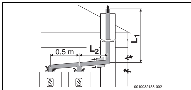
Fig. 26 Impianto a cascata con 2 apparecchi: sistema di aspirazione aria comburente/evacuazione dei prodotti della combustione rigido nel cavedio secondo B 53p con adduzione aria comburente sull'apparecchio dipendente dall'aria del locale
