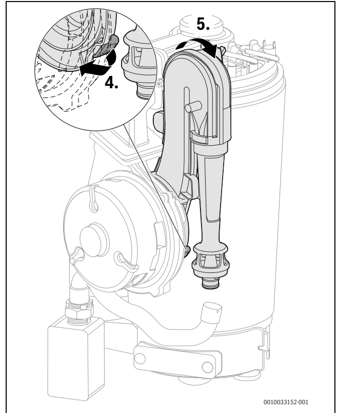
Fig. 50 Rimozione del tubo di Venturi
