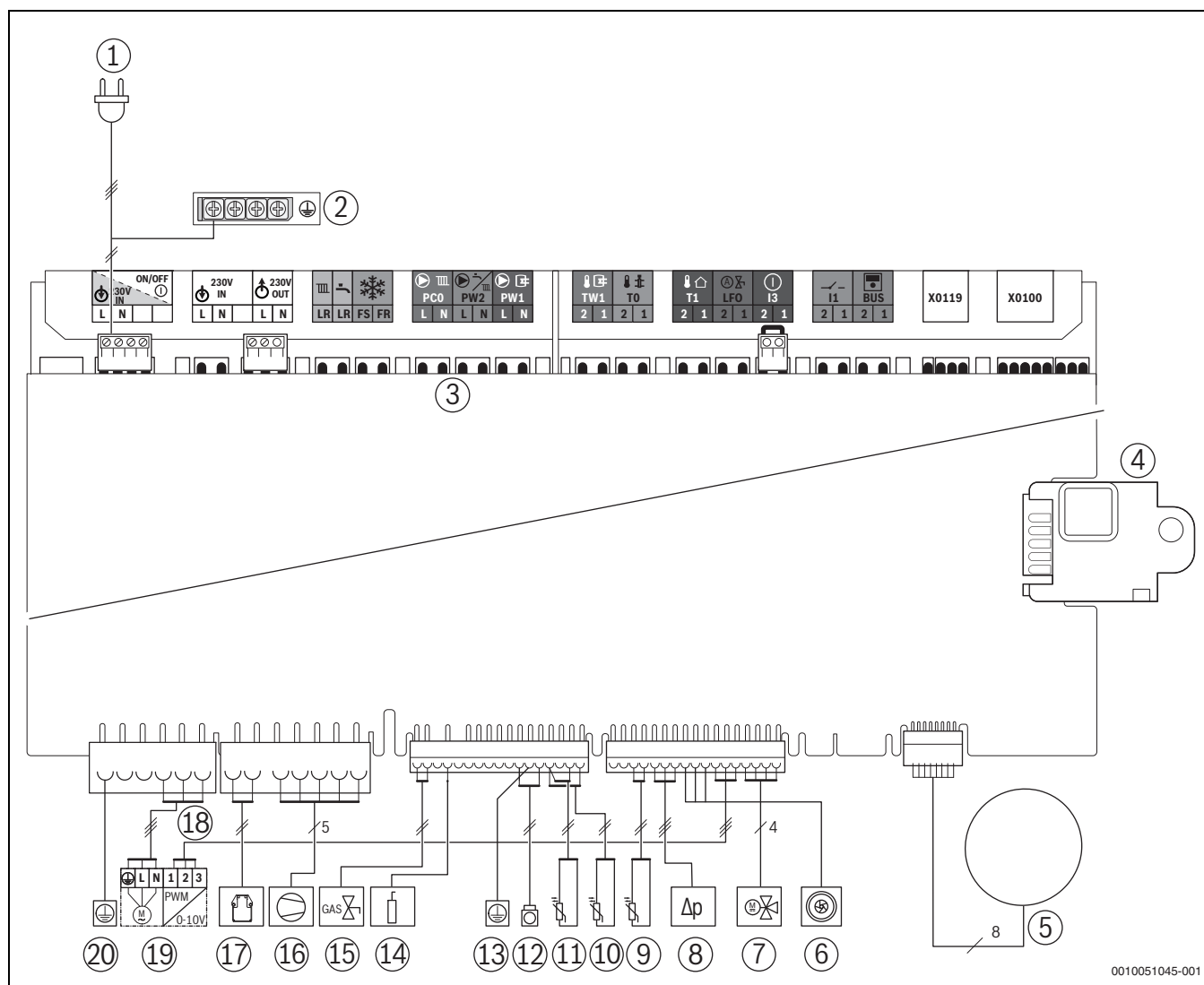
Fig. 89 Cablaggio elettrico
