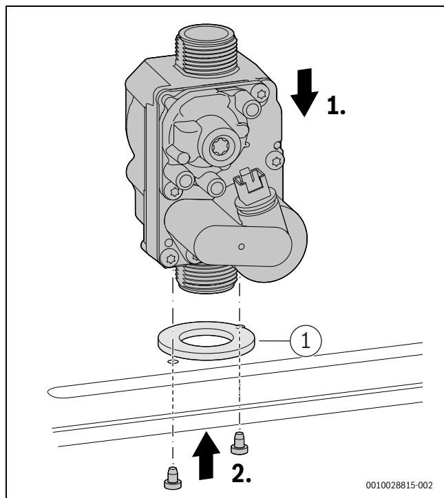
Fig. 74 Montaggio della valvola del gas
