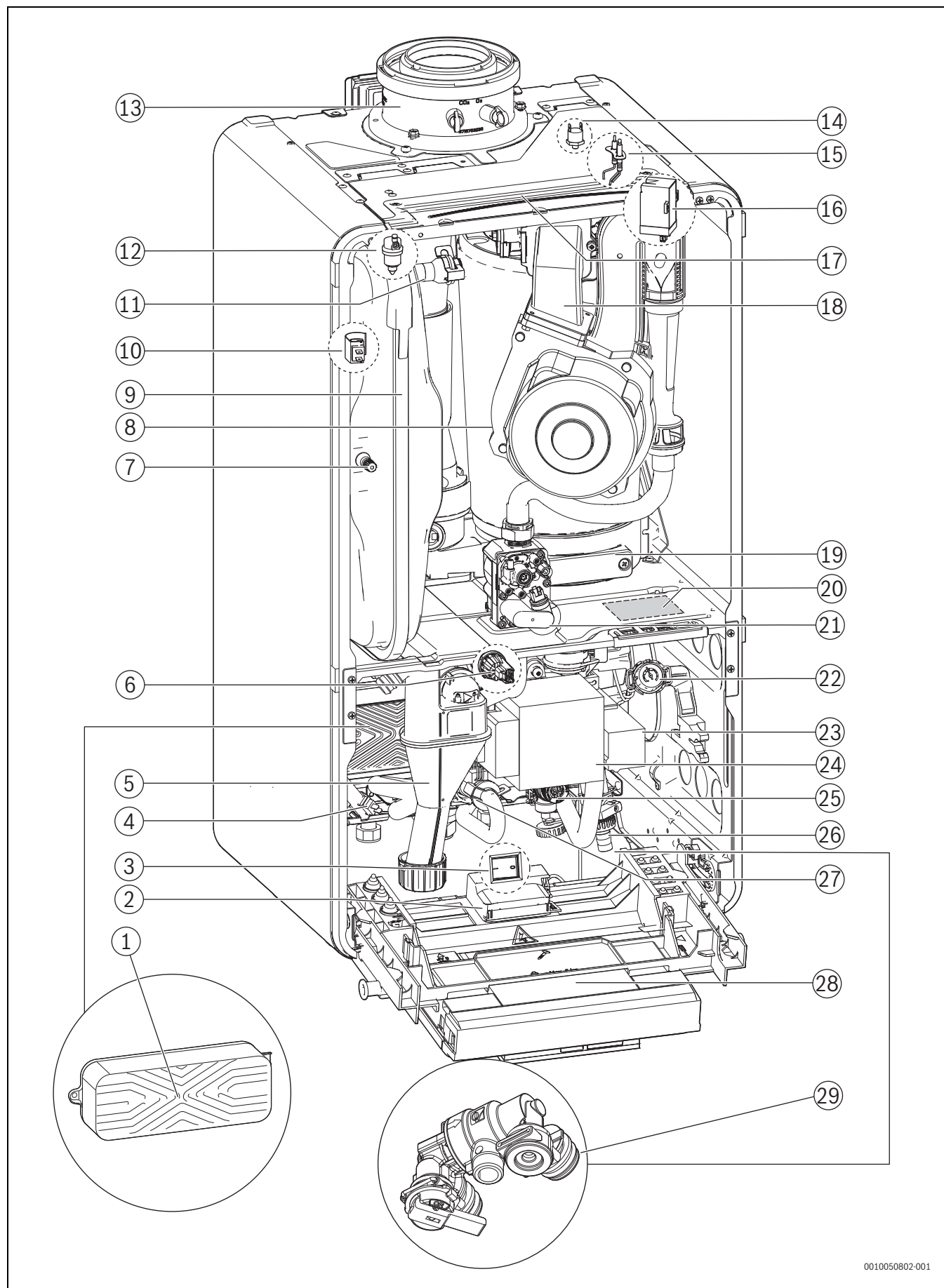
Fig. 6 Panoramica del prodotto apparecchio combi
