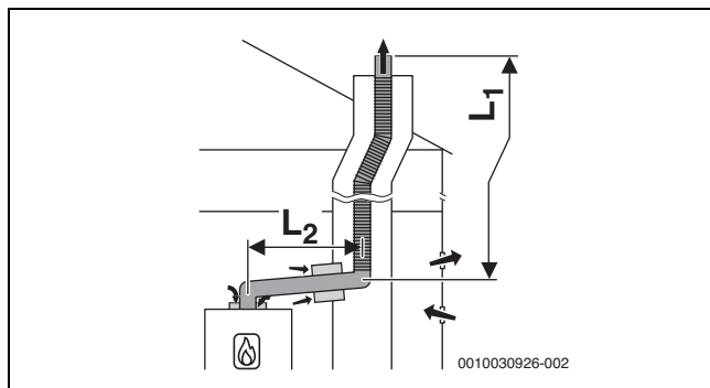
Fig. 21 Sistema fumario flessibile nel cavedio, secondo B 53p con adduzione aria comburente sull'apparecchio e dipendente dall'aria del locale e con elemento di collegamento concentrico tra luogo di posa e cavedio
