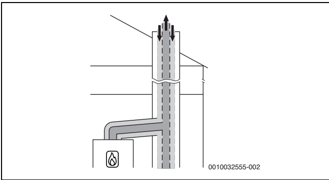
Fig. 14 Condotto di aspirazione aria comburente/evacuazione prodotti della combustione concentrico secondo C 43x nel luogo di posa
