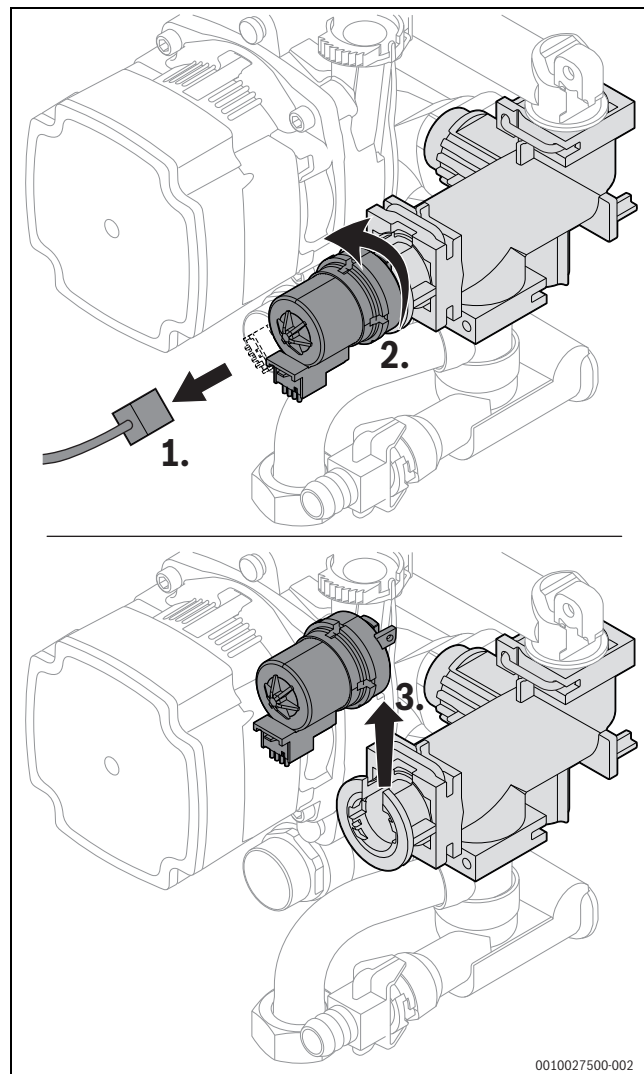
Fig. 84 Smontare il motore sulla valvola a 3 vie (variante senza viti)
