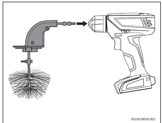
Fig. 59 Montaggio della spazzola sull'avvitatore a batteria
