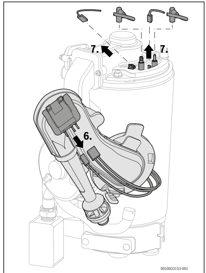
Fig. 51 Scollegamento dei cavi
