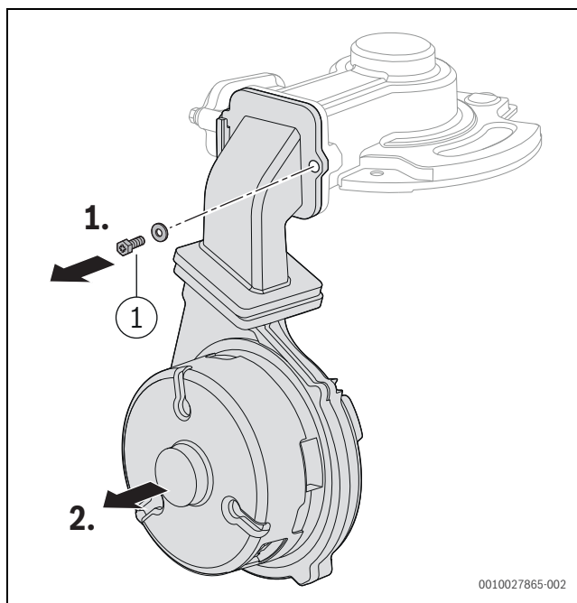
Fig. 53 Smontaggio di miscelatore e ventilatore
