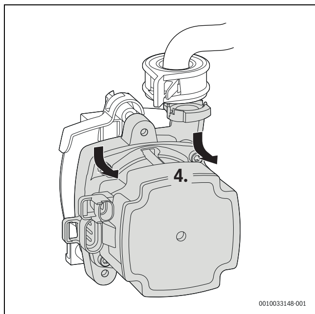
Fig. 68 Rimozione del circolatore riscaldamento
