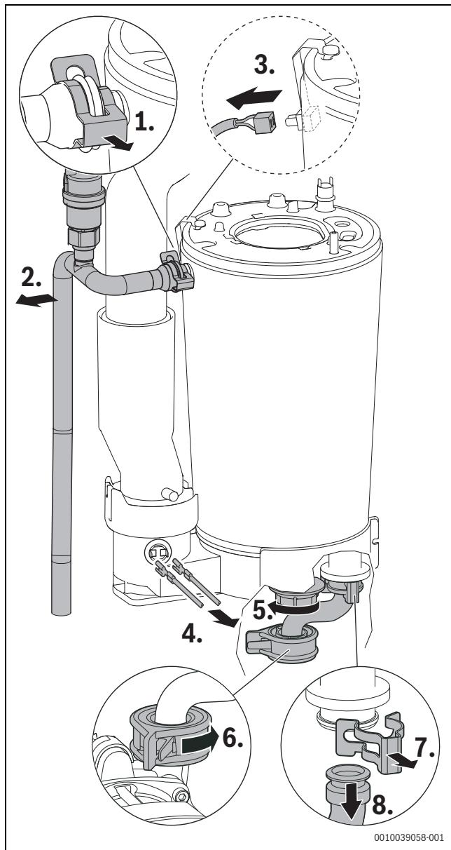
Fig. 64 Scollegamento di tubo di mandata, cavo conduttore e tubo di ritorno
