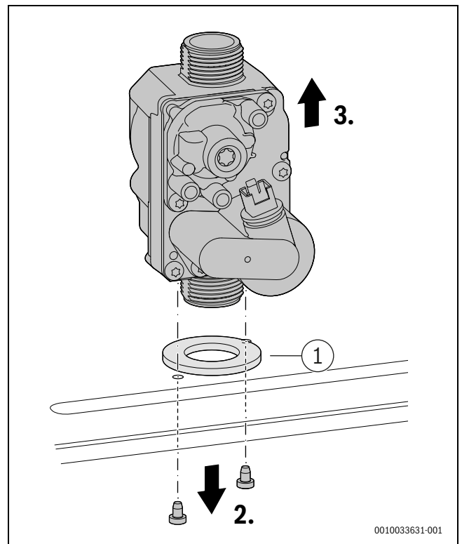
Fig. 73 Smontaggio della valvola del gas
