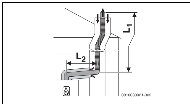
Fig. 19 Sistema di aspirazione aria comburente/evacuazione prodotti della combustione flessibile secondo C 93x nel cavedio e condotto di aspirazione aria comburente/evacuazione prodotti della combustione concentrico nel luogo di posa
