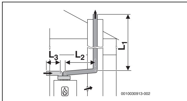
Fig. 15 Sistema di aspirazione aria/evacuazione pdc rigido secondo C53 nel cavedio e condotto di aspirazione aria comburente/evacuazione pdc con tubi separati per adduzione aria ed evacuazione pdc nel luogo di posa
