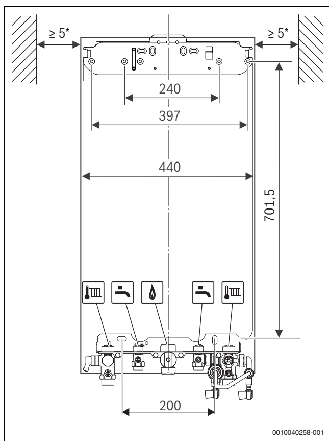
Fig. 3 Vista anteriore (mm)
