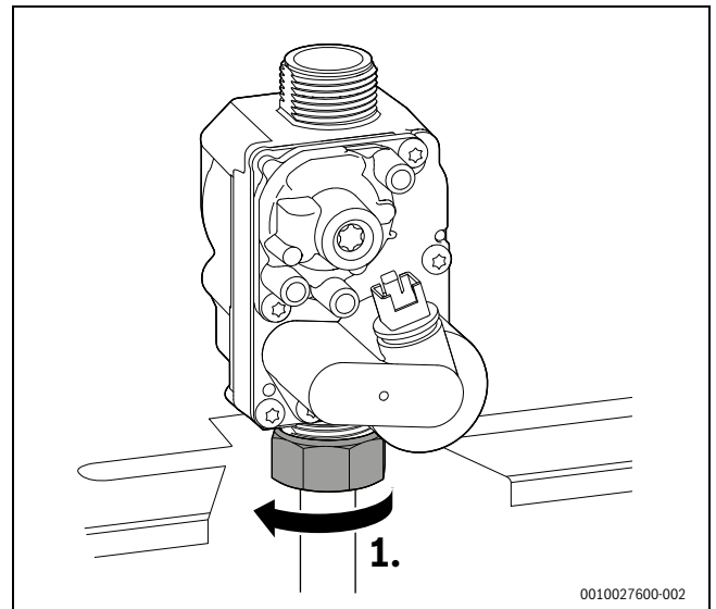
Fig. 72 Svitamento del dado a risvolto
