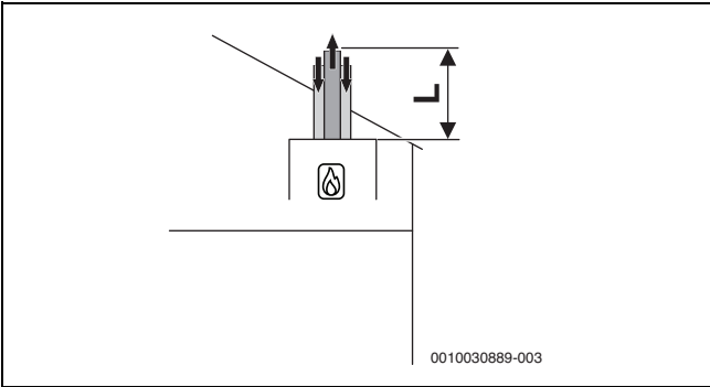
Fig. 13 Condotto di aspirazione aria comburente/evacuazione prodotti della combustione verticale concentrico secondo C 33x
