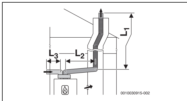
Fig. 16 Sistema di aspirazione aria/evacuazione prodotti della combustione flessibile secondo C53 nel cavedio e condotto di aspirazione aria comburente/evacuazione pdc con tubi separati per adduzione aria ed evacuazione pdc nel luogo di posa
