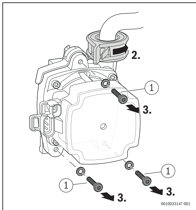
Fig. 67 Sbloccaggio del circolatore riscaldamento e rimozione delle viti
