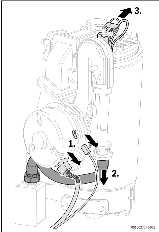
Fig. 49 Scollegamento di connettore elettrodi d'accensione e tubo flessibile del gas
