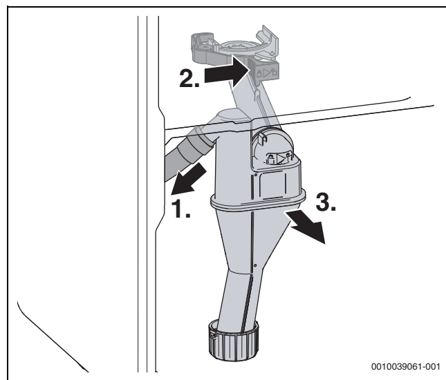
Fig. 79 Smontaggio del sifone per la condensa
