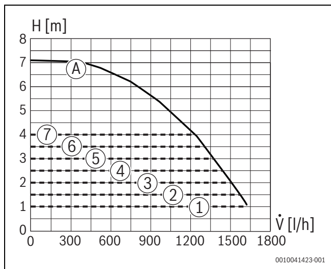
Fig. 88 Campi di lavoro del circolatore e relative curve caratteristiche
