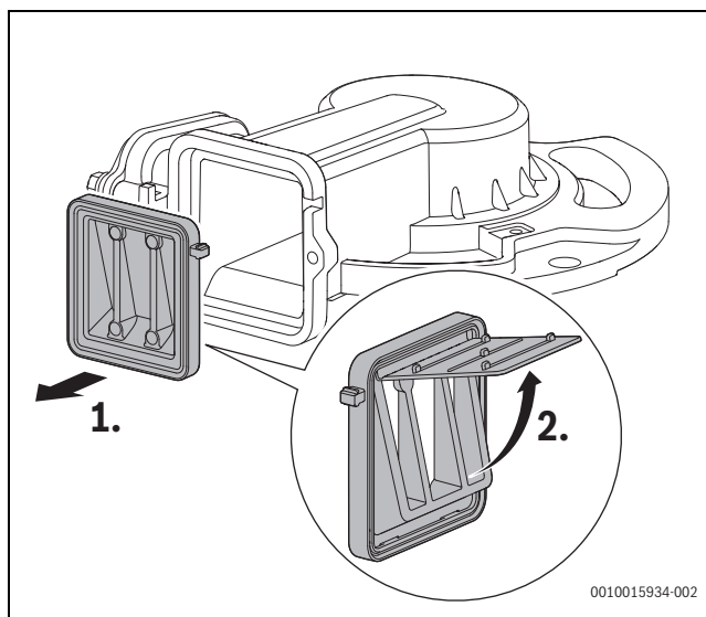
Fig. 54 Protezione antiriflusso nel miscelatore
