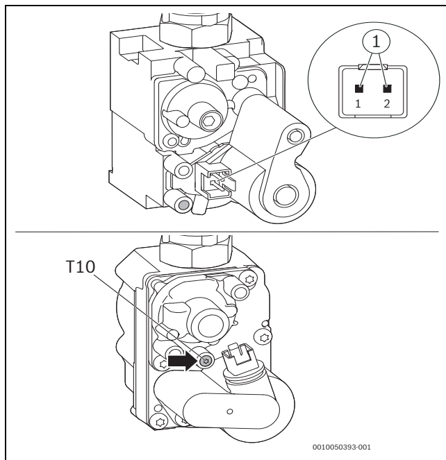
Fig. 48 Punti di misurazione sulla valvola del gas
